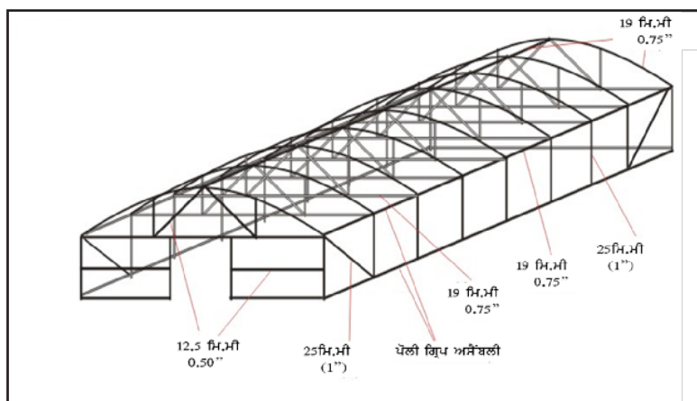
ਚਿੱਤਰ 2 : ਪੌਲੀਨੈੱਟ ਹਾਊਸ ਵਿੱਚ ਵਰਤੀਆਂ ਗਈਆਂ ਪਾਈਪਾਂ ਦਾ ਵਿਵਰਣ (62.5 ਮੀਟਰ x 8.0 ਮੀਟਰ)
